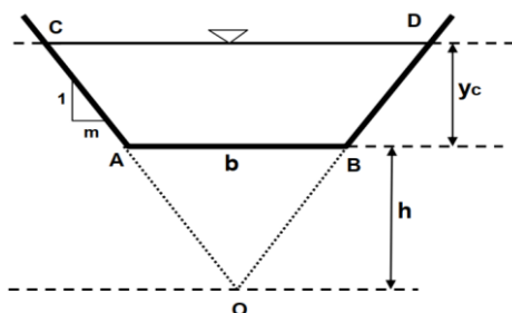
شکل ۱- پارامترهای هندسی و هیدرولیکی در مقطع بحرانی Fig 1. Geometric and hydraulic parameters at the critical section
