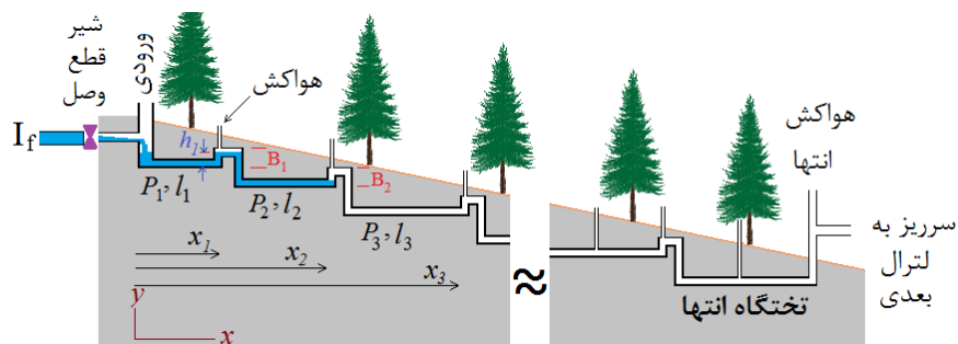
شکل ۲- شماتیک جانبی وضعیت قرارگیری تخته‌گاه‌ها ( P_1 و P_2 و ..) و موانع ( B_1 و B_2 و ..) در طول لترال.
