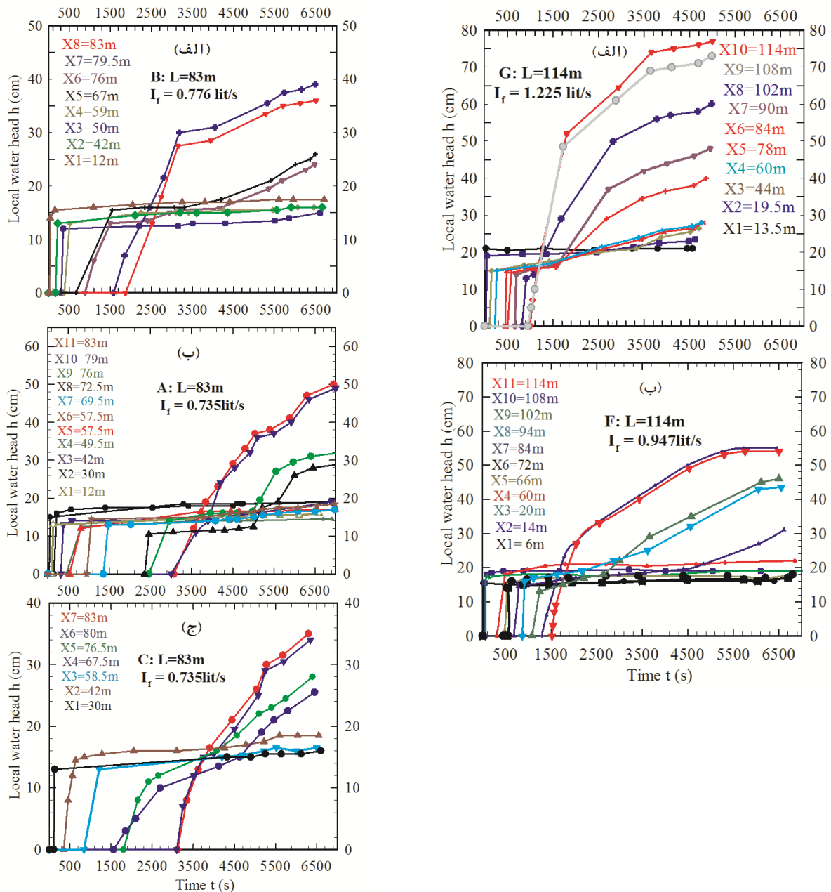
شکل ۴- تغییرات زمانی هد آب در تخته‌گاه‌های دو لترال با طول یکسان و (الف) دبی ۱/۲۲۵ و (ب) دبی ۰/۹۴۷ لیتر بر ثانیه.
