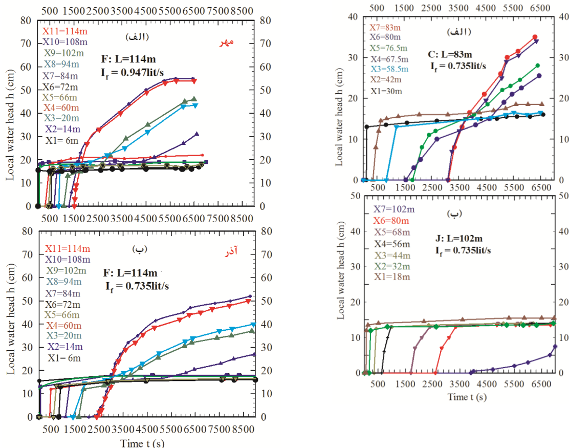
شکل ۶ - تغییرات زمانی هد آب در تخته‌گاه‌های دو لترال با دبی ۰/۷۳۵ لیتر بر ثانیه و طول‌های، الف) ۸۳ متر و ب) ۱۰۲ متر در دو زمان از سال، الف) مهر و ب) آذر. شکل ۷ - تغییرات زمانی هد آب در تخته‌گاه‌های لترال F که دارای ۹ تخته‌گاه و ۸ مانع سیفون‌گونه است، در دو زمان متفاوت از سال (مهر و آذرماه) را نشان می‌دهد. همانطور که قبلاً اشاره شد، تراوایی این سیستم زیرسطحی به درصد رطوبت اولیه خاک نیز بستگی دارد. در مهر ماه که تابش خورشید بیش از آذر است، میزان جذب آب توسط درختان بمراتب بیش از آذر ماه و به تبع میزان رطوبت خاک کمتر بوده و در نتیجه متوسط تراوایی لترال بیشتر و لذا از دبی آب ورودی بیشتری در فرایند آبیاری استفاده شد، بر عکس، در آذر ماه علیرغم اینکه دور آبیاری طولانی ۴۰ روز بود، رطوبت نسبی خاک بیشتر، و دبی لازم برای آبیاری کمتر (۰/۷۳۵ لیتر بر ثانیه) کفایت می‌کند. از مقایسه تغییرات زمانی هد تخته‌گاه‌های ابتدای خط، در می‌یابیم که با کاهش دبی آب ورودی به لترال، هد آب در تخته‌گاه‌های ابتدای خط نیز کاهش می‌یابد که این پدیده ناشی از کاهش مقاومت جریان در اثر عبور آب از دو خم بالای هر مانع می‌باشد. از این آزمون‌ها نتیجه می‌گیریم که دبی بهینه و لازم برای آبیاری لترال نه تنها به طول آن بستگی دارد بلکه به زمان (از سال) انجام فرایند آبیاری نیز بستگی دارد.
