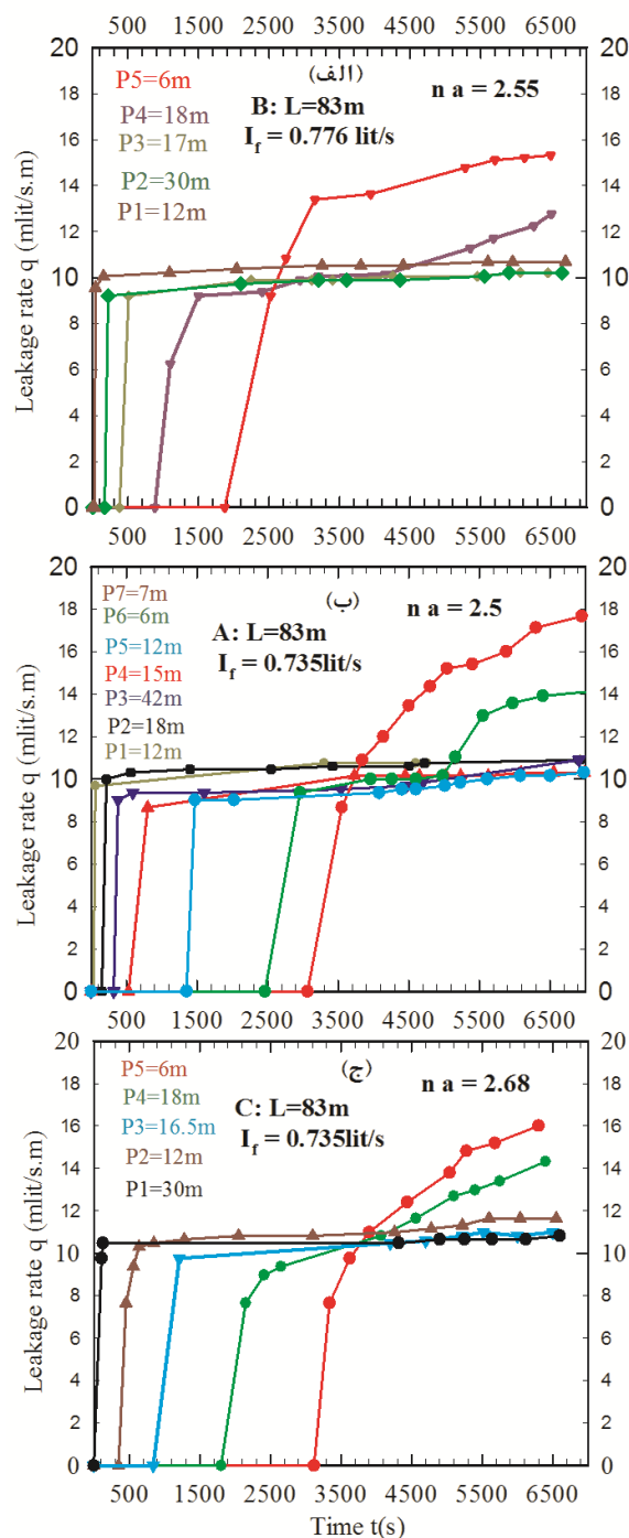
شکل ۹ - نتایج شبیه‌سازی تغییرات زمانی تراوایی واحد طول q درختگاه‌های سه لترال با طول یکسان و الف) دبی ۰/۷۷۶ (ب) دبی ۰/۷۳۵ (ج) ۰/۷۳۵ لیتر بر ثانیه (ممتناظر با نتایج تجربی شکل ۵).
