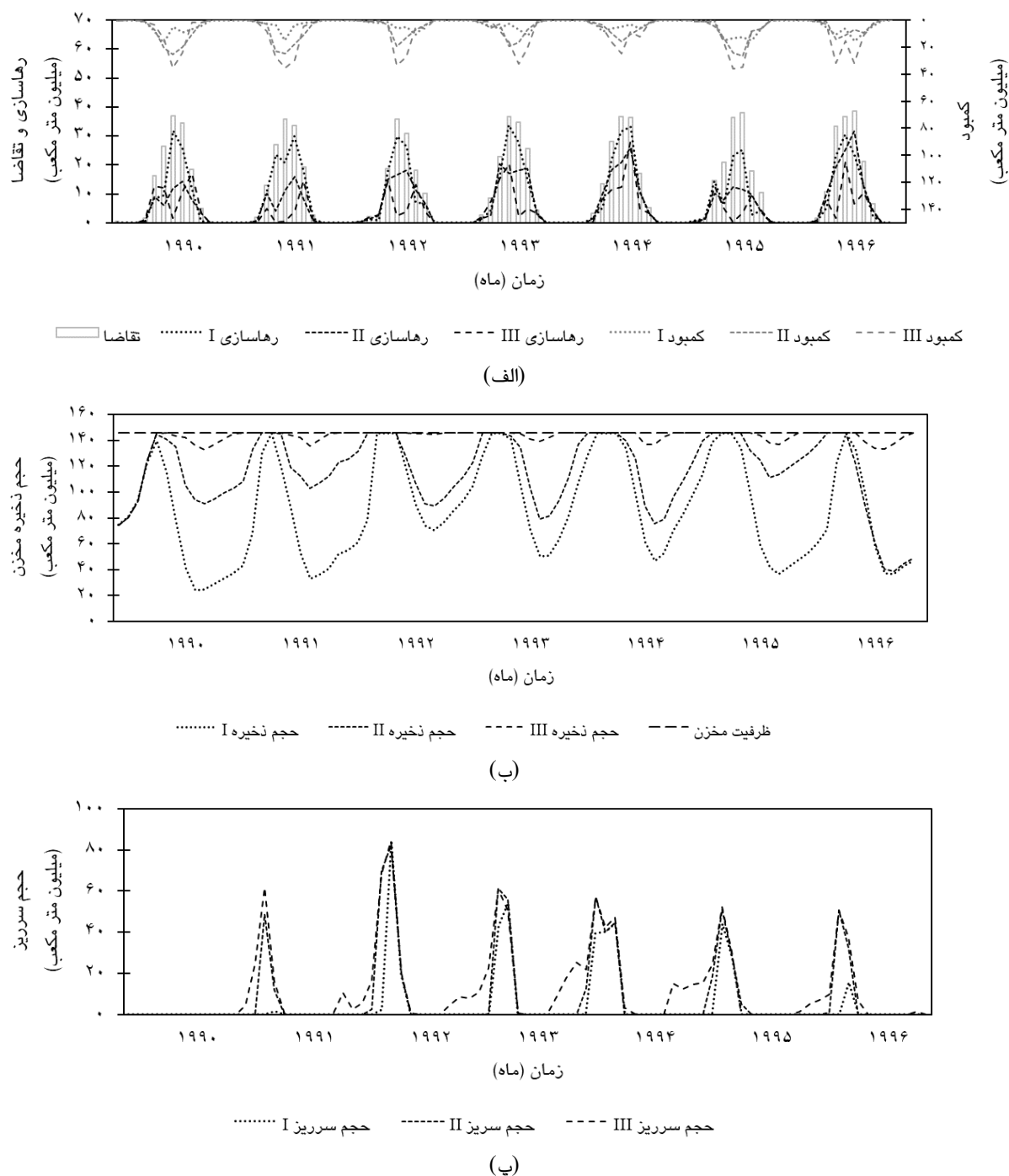
شکل ۶- نمایش (الف) رهاسازی و تقاضا، (ب) حجم ذخیره مخزن و (پ) سرریز از مخزن آیدوغموش برای سه سیاست I، II و III در بازه ۷ ساله (۱۹۹۰-۱۹۹۶).
